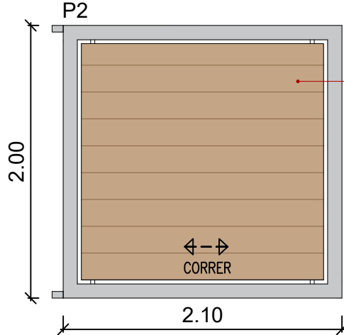
Detalhe – Porteira de correr escala + 1/40
