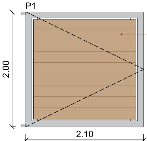
Detalhe – Porteira de abrir escala + 1/40
