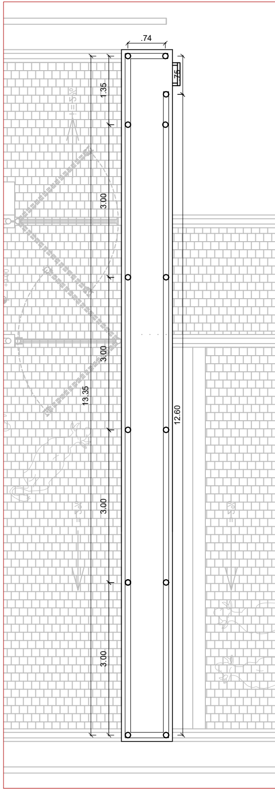
Planta Baixa – Plataforma de Observação escala + 1/75
